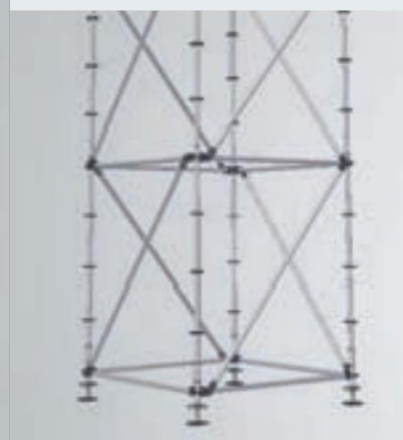
Schema tipo per torre con carico ammissibile di 30 kN per stelo
