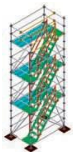
Scala a torre monodirezionale
